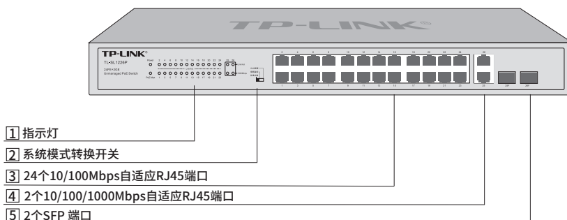
图1-4 TL-SL1226P前面板示意图
