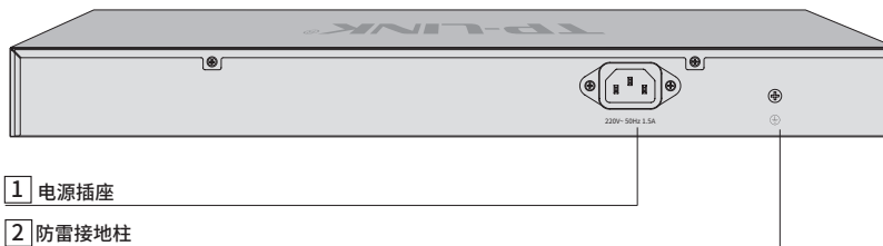
图1-7 TL-SL1218PE-Combo后面板示意图
